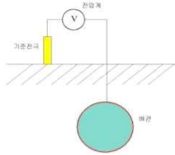
[그림 11.2] 매설배관의 방식전위 측정 개념도
